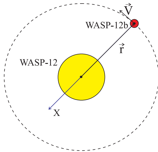
Рис. 1. К определению орбиты экзопланеты WASP-12b.
